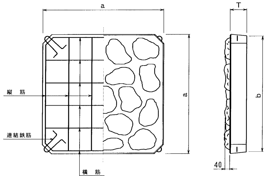
形状図
