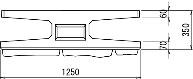
平面図
