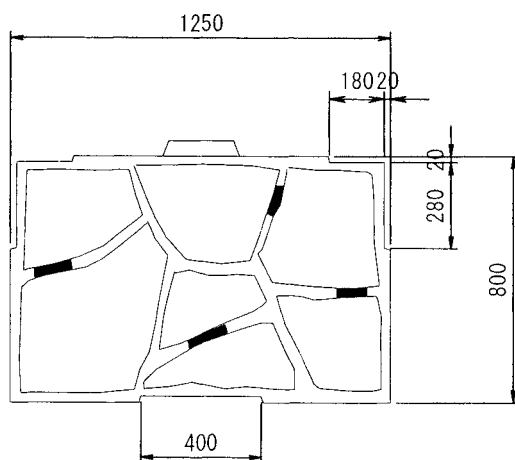
正面図
