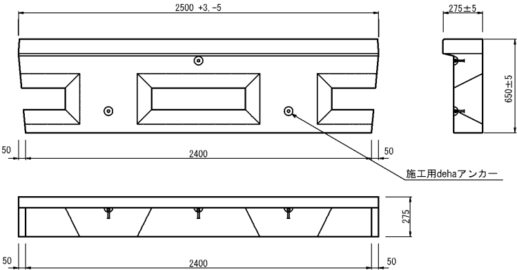
参考：基礎ブロック
