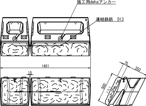
参考：基礎ブロック
