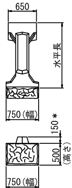
D形(端部1/2)
