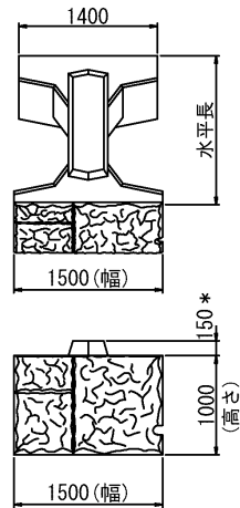
A形(基本)
