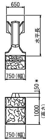
B形(端部)
