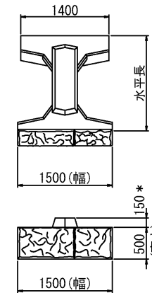
C形(基本1/2)
