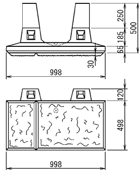
A形 (天端)
