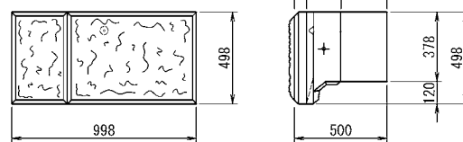
A形 (水抜)
