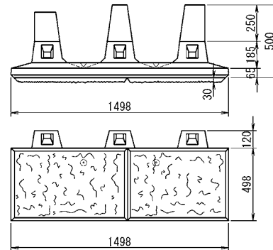
C形 (根石)
