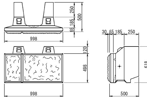
C形 (根石)
