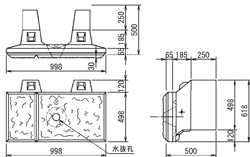
A形 (水抜)
