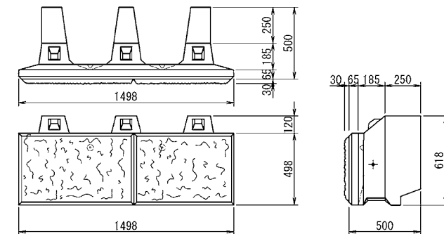
F形 (根石端部)
