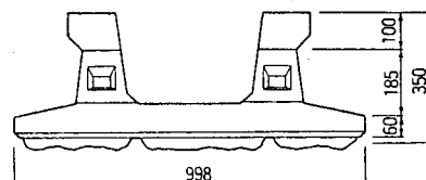
A形(基本)
