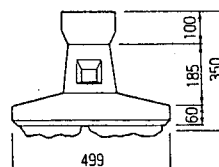
B形(端部)
