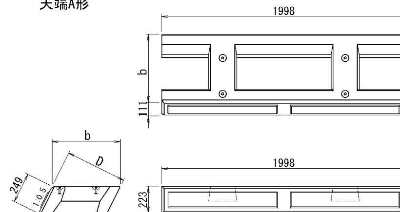
天端A形
