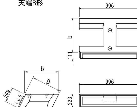
天端B形
