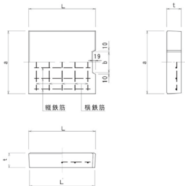
形状及び配筋
