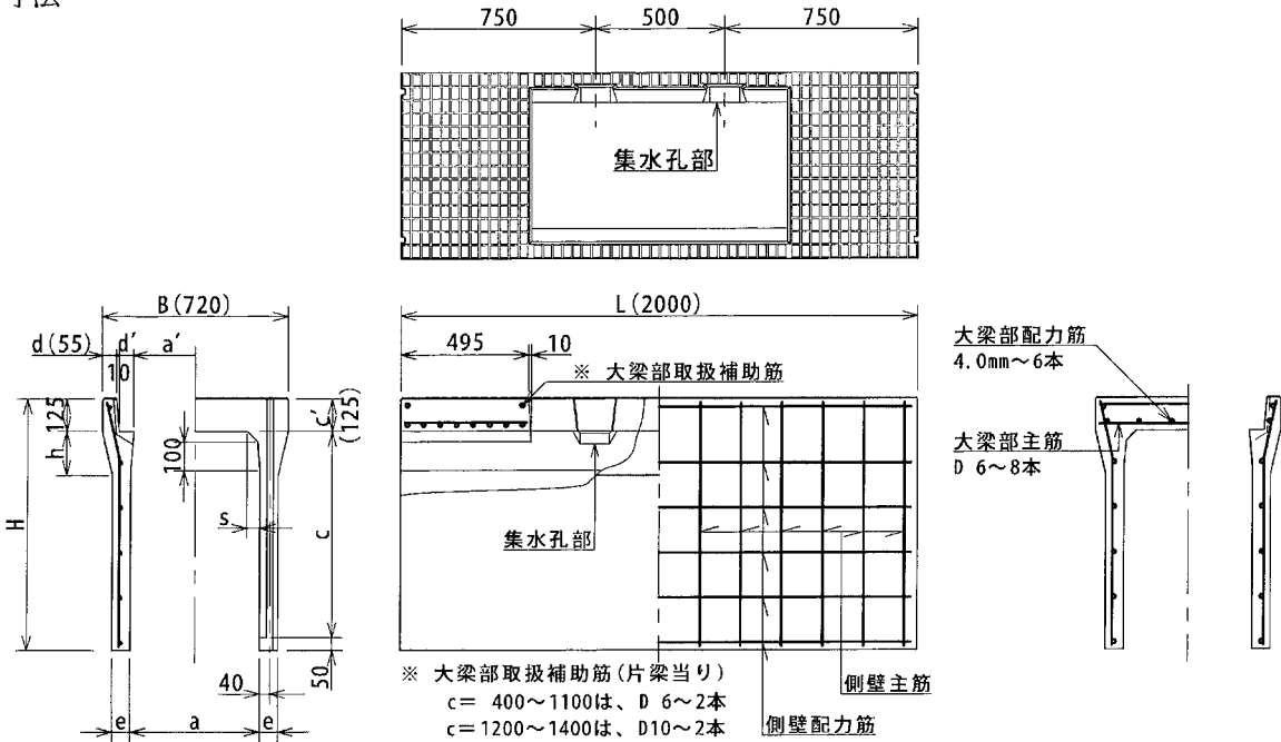
形状寸法
