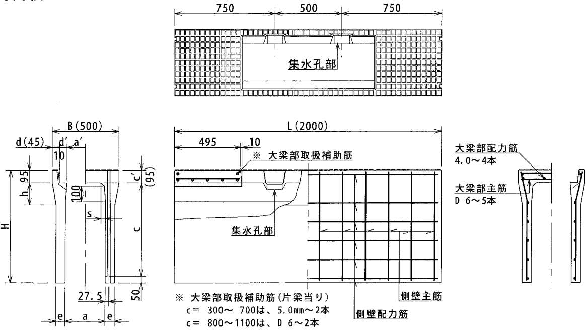
形状寸法
