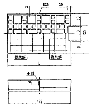
蓋板寸法及び配筋表
