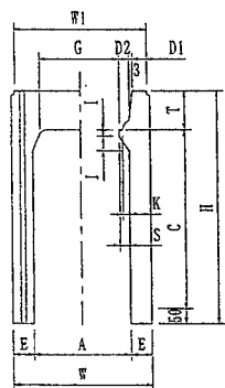
寸法及び配筋表
