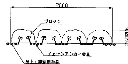
正面図
