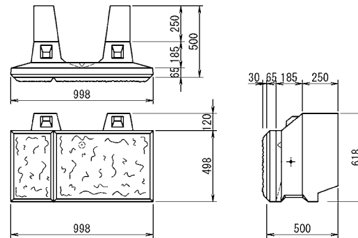
C形(根石)
