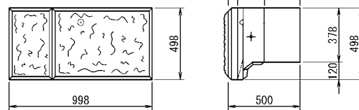
A形(水抜)
