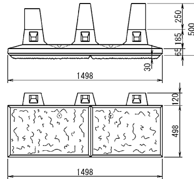
C形(根石)
