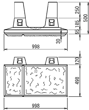
A形(天端)
