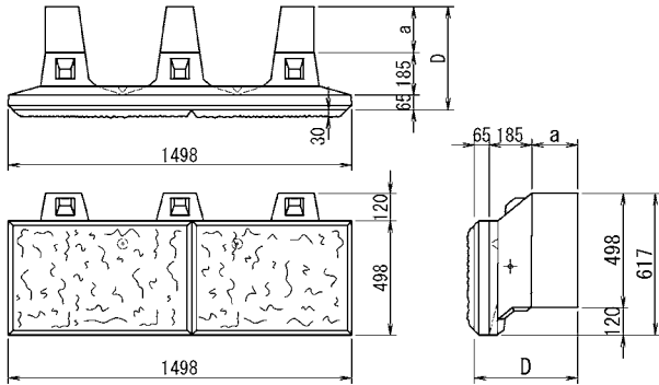
C形 (根石)
