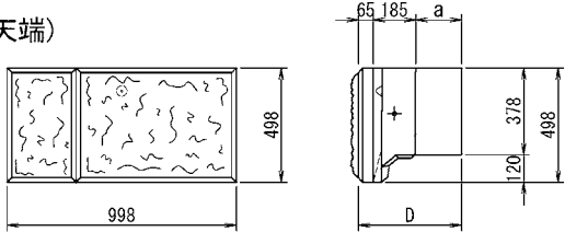
A形 (水抜)
