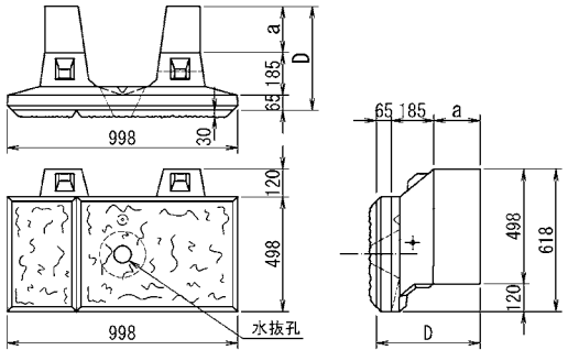
A形 (水抜)
