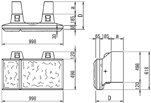
A形 (天端)
