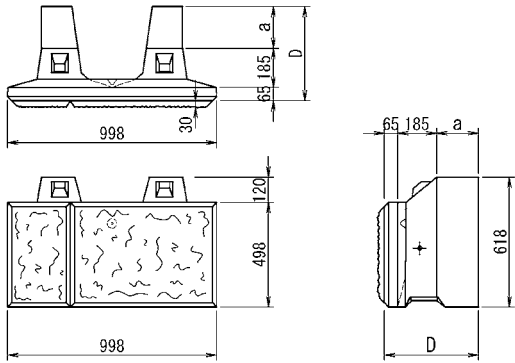
C形 (根石)
