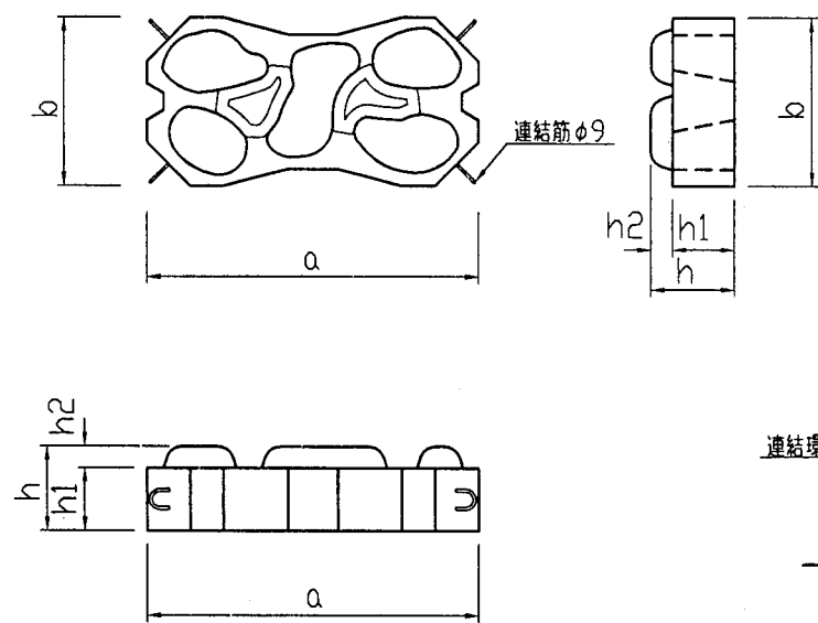
連結部詳細図
