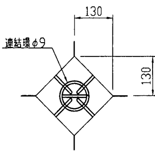
連結部詳細図
