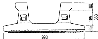
A形(基本)
