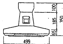
B形(端部)
