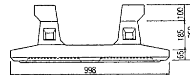
C形(根石)
