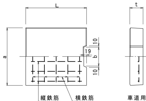
形状及び配筋
