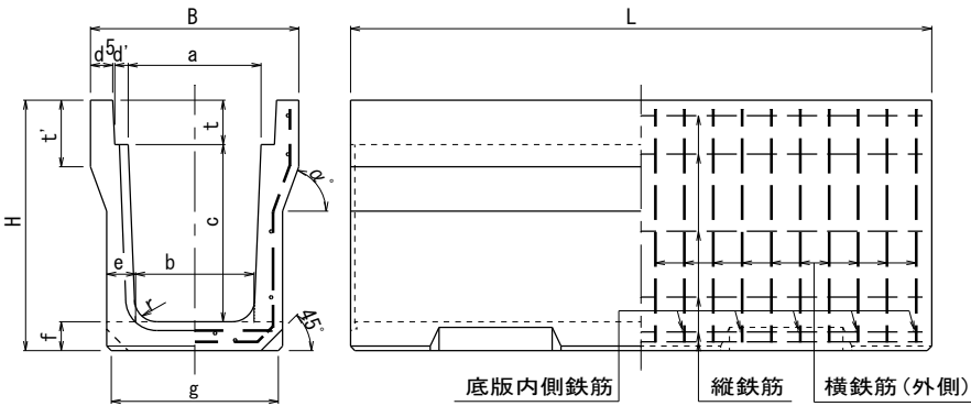
形状及び配筋
