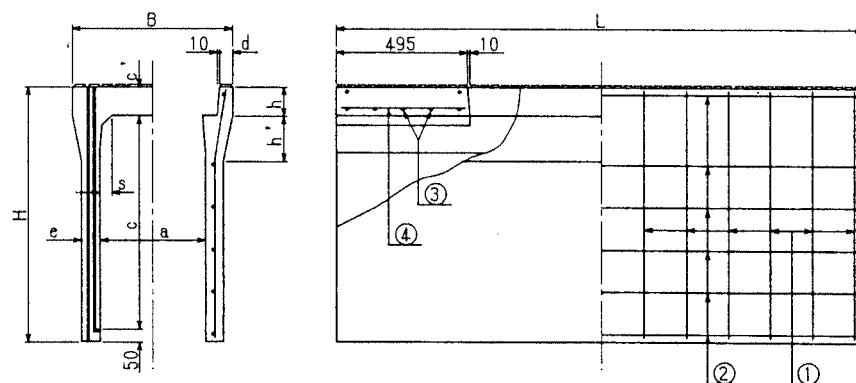
寸法及び配筋表
