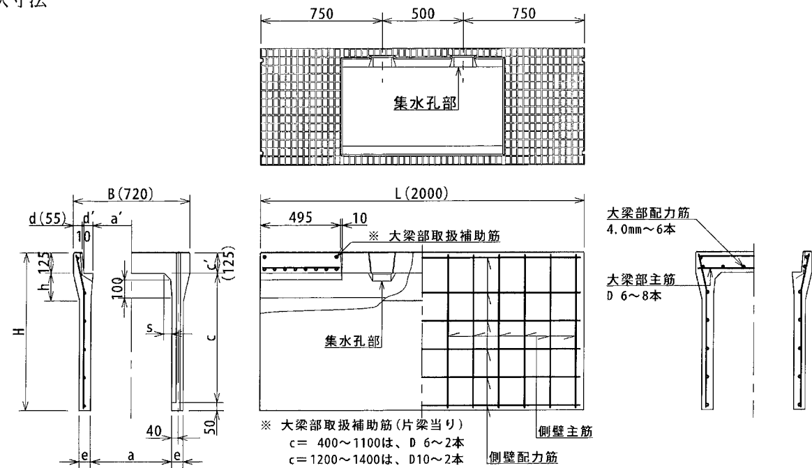
形状寸法
