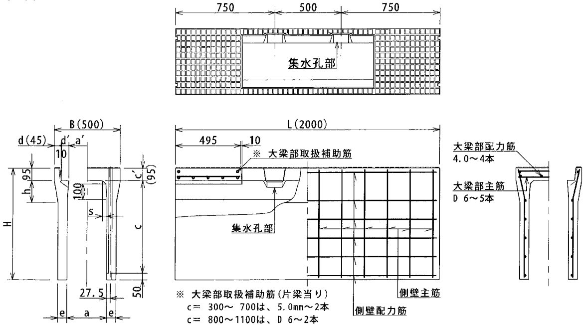
形状寸法
