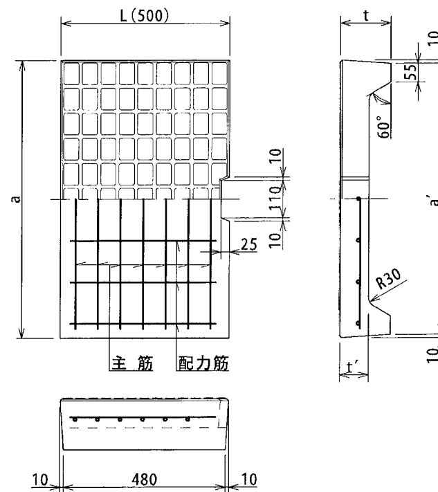
● 寸法・配筋表
