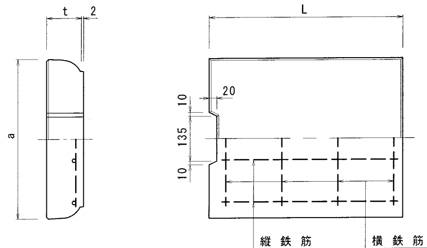
形状及び配筋図
