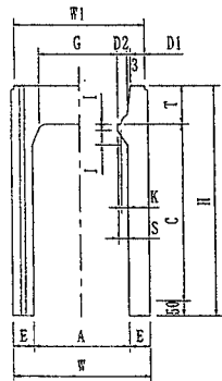
寸法及び配筋表
